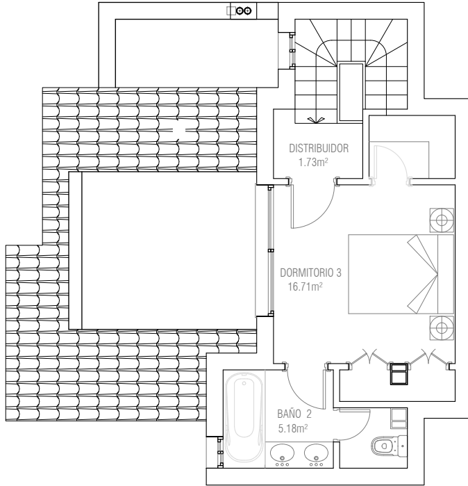
PLANTA ÁTICO
