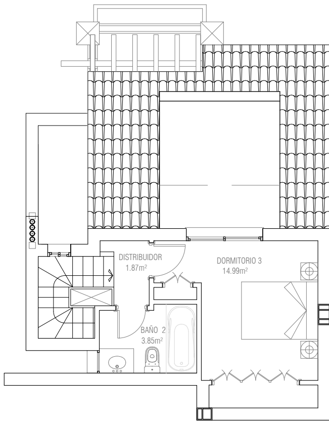
PLANTA ÁTICO
